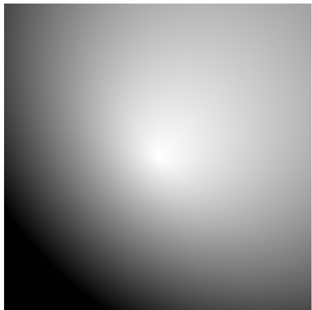
RadialGradient()
